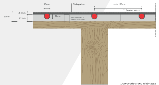
Doorsnede Mono gietmassa
