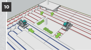
Zaag de eerste dekplaat op maat en plaats in de hoek
