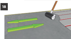
18 Rol direct de gietmassa door met een prikkroller
