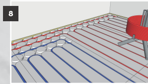
Leg de buis volgens de gewenste groep indeling
