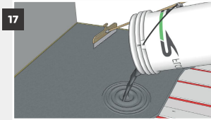
17 Giet de gietmassa over de vloer en breng op hoogte met een rakel
