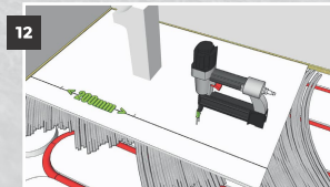
Plaats de eerste plaat in de lijm en niet vast met spreidnieten
