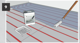
De vloer voorbehandelen met Multiprimer
