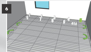
Plaats alle elementen per rij en volgens de buisindeling
