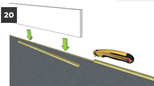
20 Kantstroken wegsnijden en plinten plaatsen
