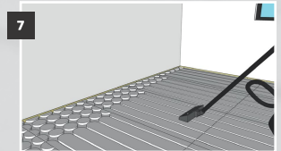
De vloer grondig stofzuigen zodat de sleuven stof vrij zijn
